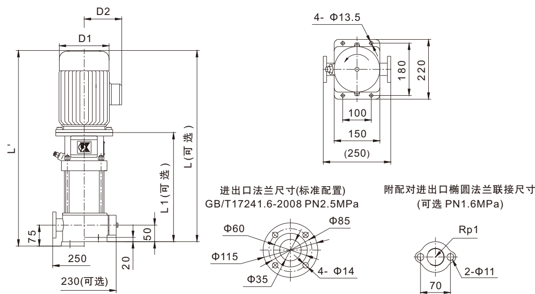
KQDP25-2
