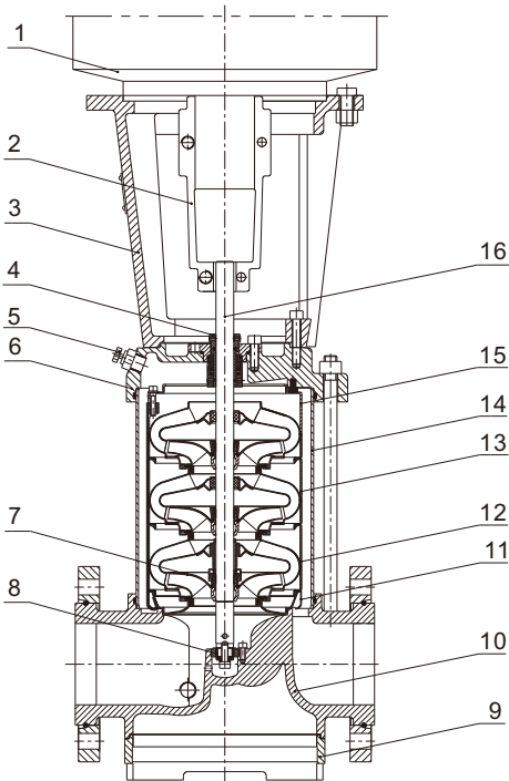
KQDQ80-45、100-64、100-90
