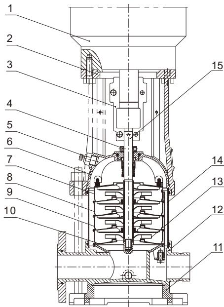
KQDQ40-8、40-10、50-12
