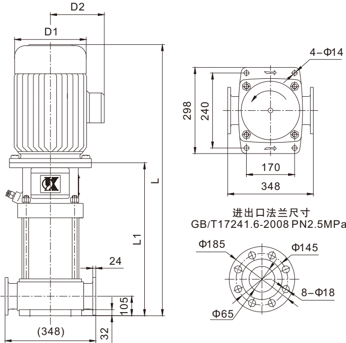
KQDP65-32
