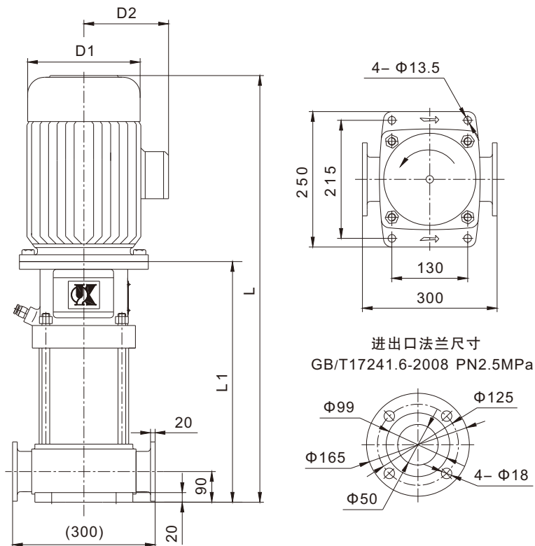
安装图
