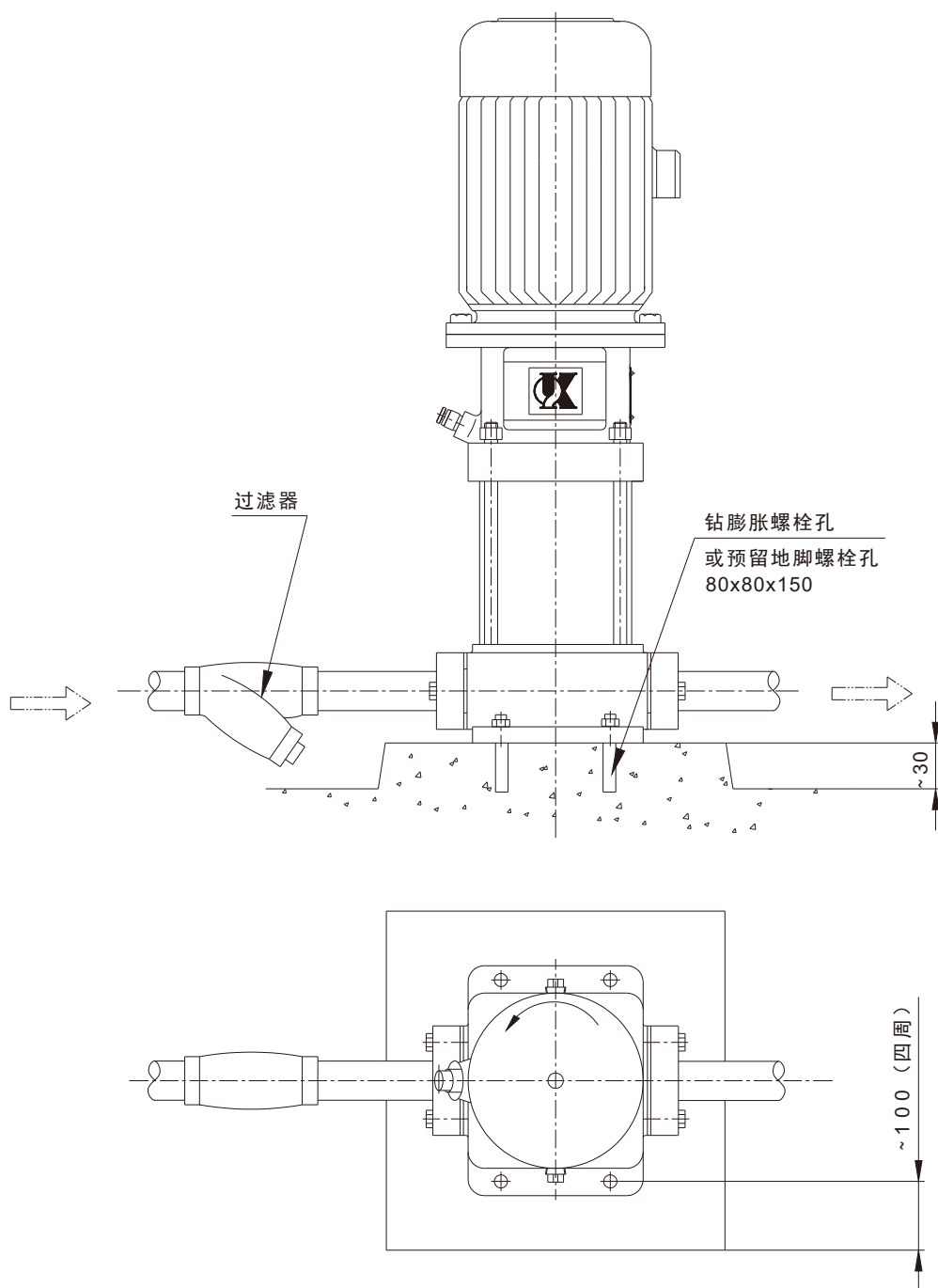
KQDP、KQDQ 安装图
