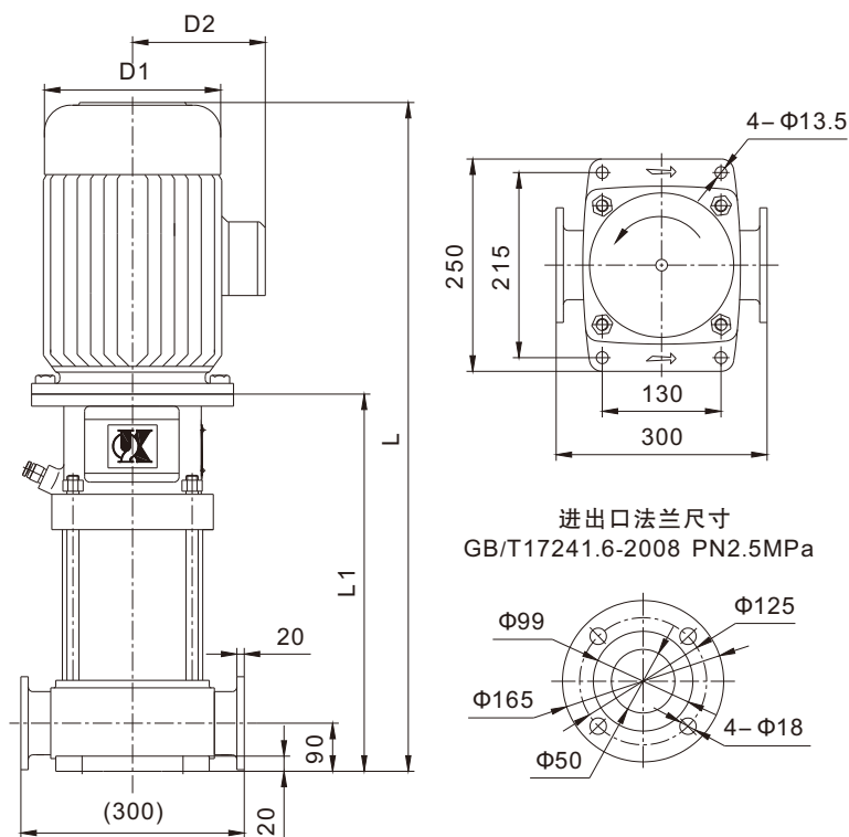
安装图
