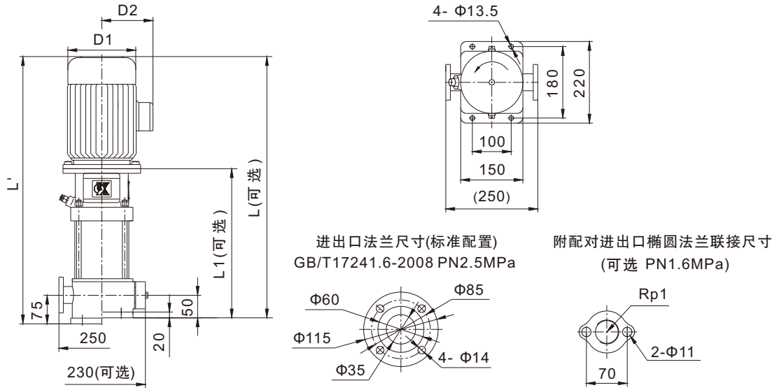
安装图
