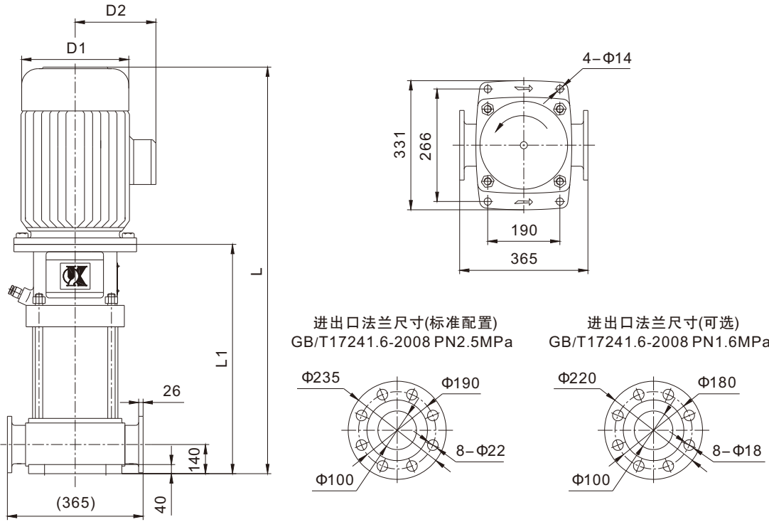
安装图
