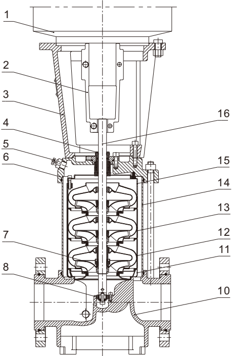
KQDP80-45、100-64、100-90
