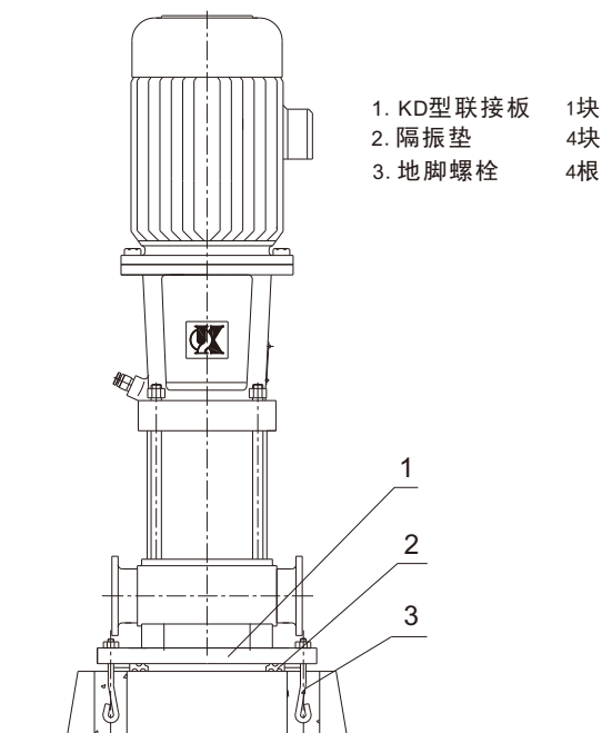
柔性连接（隔振垫）
