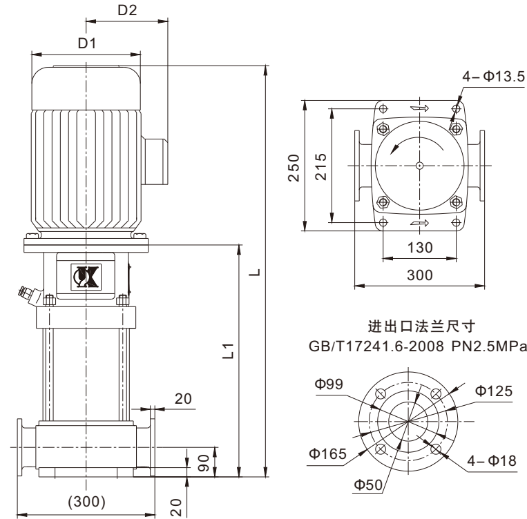
安装图
