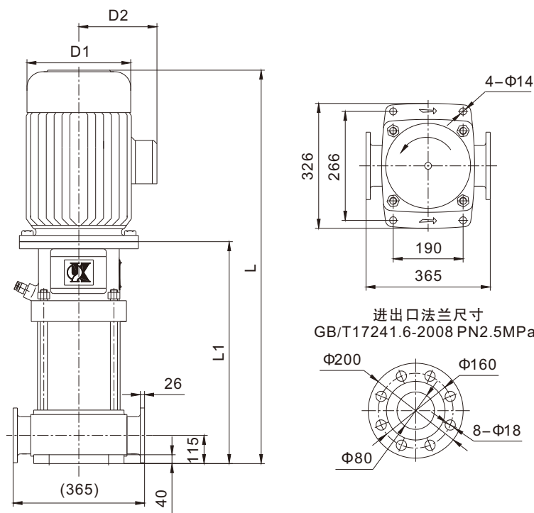
KQDP80-45
