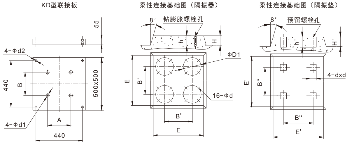
柔性安装基础尺寸图
