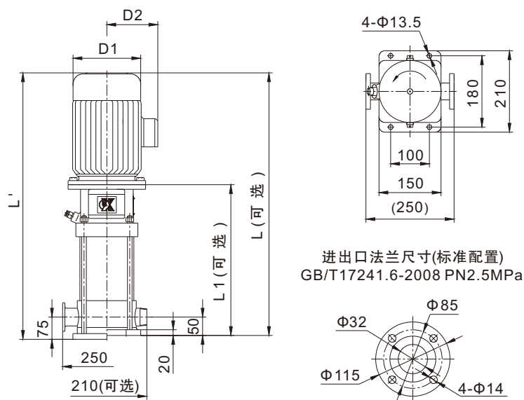
KQDQ25-1
