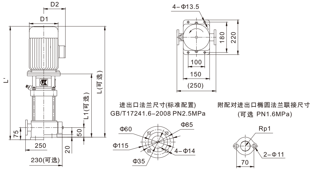
KQDP25-1
