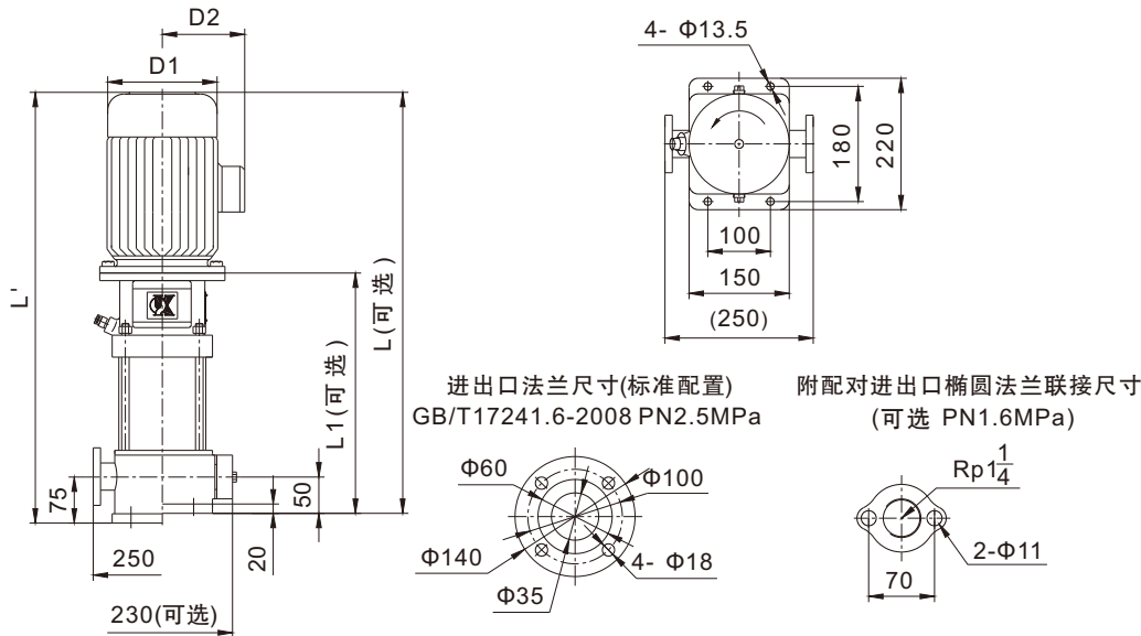
KQDP32-5
