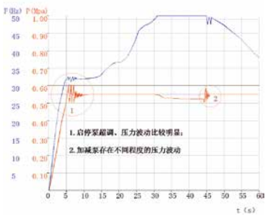
普通单变频性能曲线
