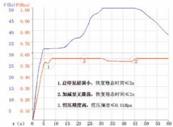
数字全变频性能曲线
