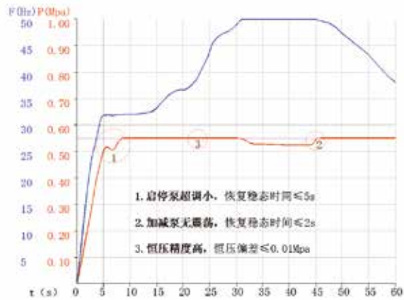
数字全变频性能曲线
