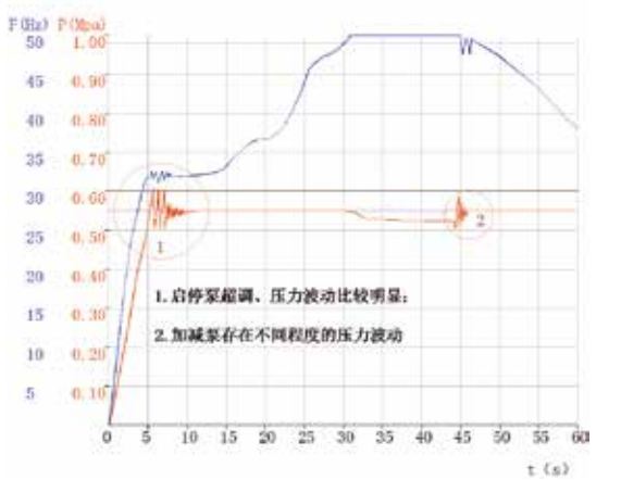
普通单变频性能曲线
