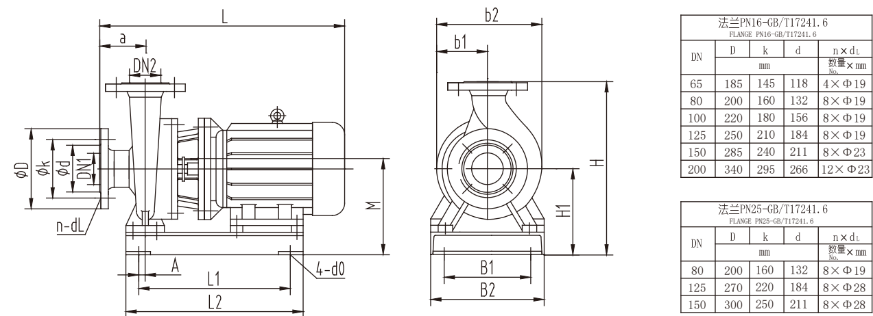
卧式安装尺寸图
