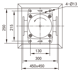
进出口法兰尺寸
