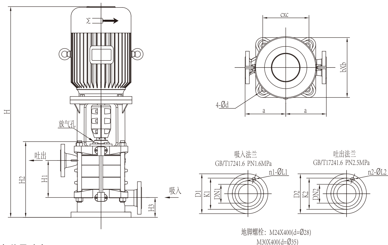
安装尺寸表
