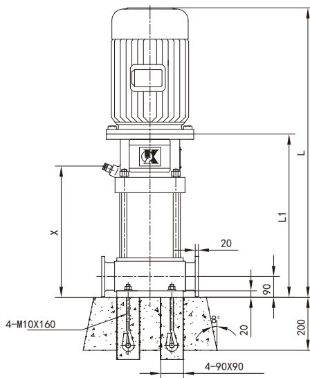
安装尺寸图
