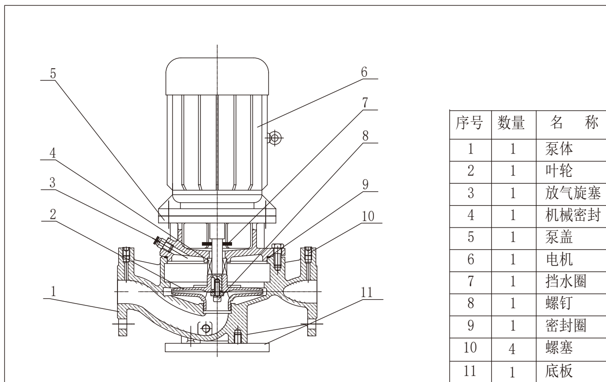
立式单级/第五代XBD系列立式单级电动机消防泵组结构图
