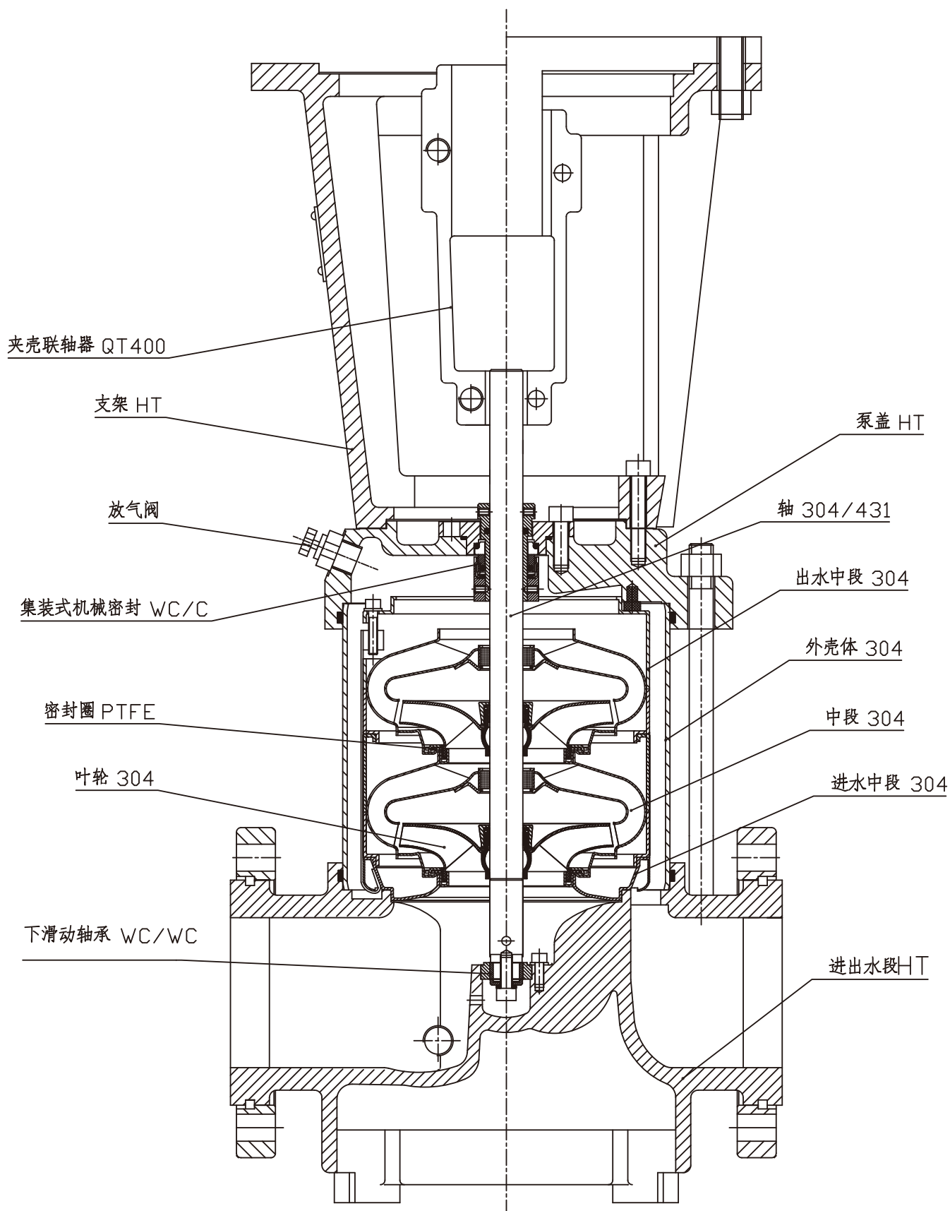
XBD-65、80、100DP结构图
