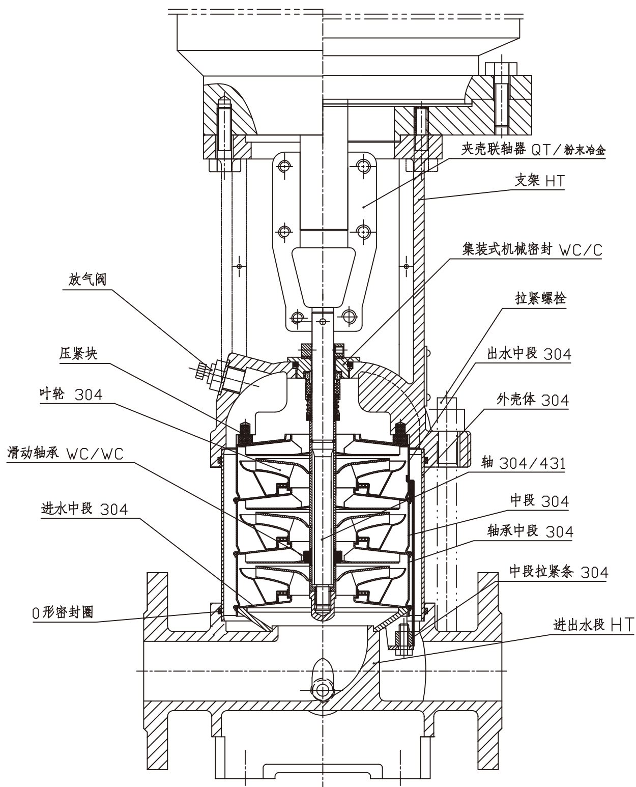
XBD-40、50DP结构图
